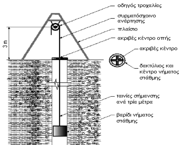
Σχήμα 2 - Διάταξη ελέγχου κατακόρυφης υδρογέωτρησης
